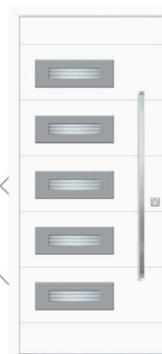
Model BASEL RAL boja 9016 MAT Staklo DPL Aplikacije float kaljene/emajlirane RAL 9006 Rukohvat KCR 115h Rozeta RPP 50
