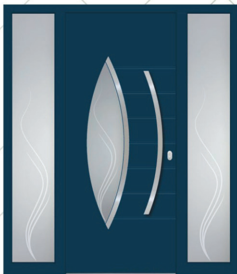
Model ATHENS RAL boja 5001 Staklo DPG Aplikacija POLIRANA Rukohvat POA 115h Rozeta ROP 50 Dosljetlo lijevo i desno DPG
